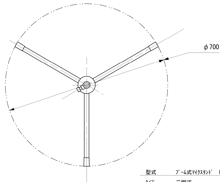
A-A'' 矢视图
