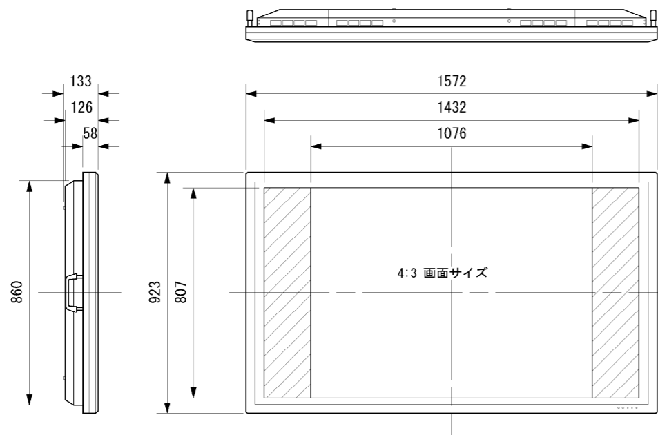
液晶ディスプレイ SHARP PN-G655 (S=1:20)
