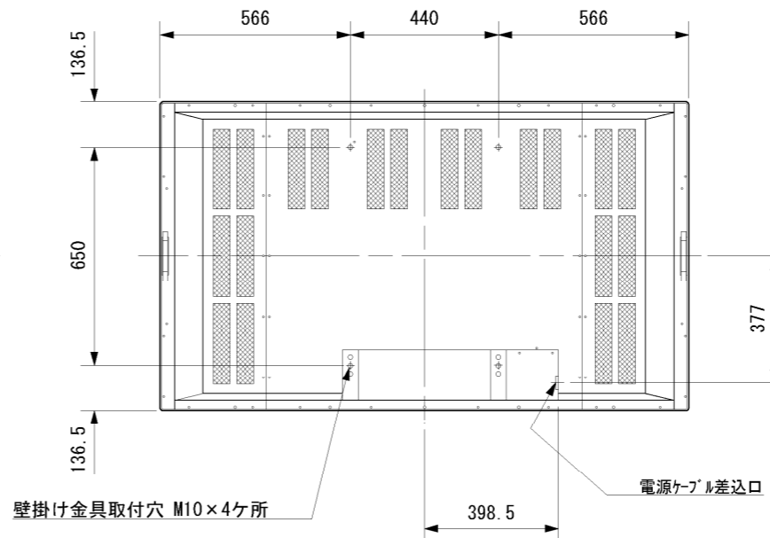
液晶ディスプレイ SHARP PN-G655 (S=1:20)
