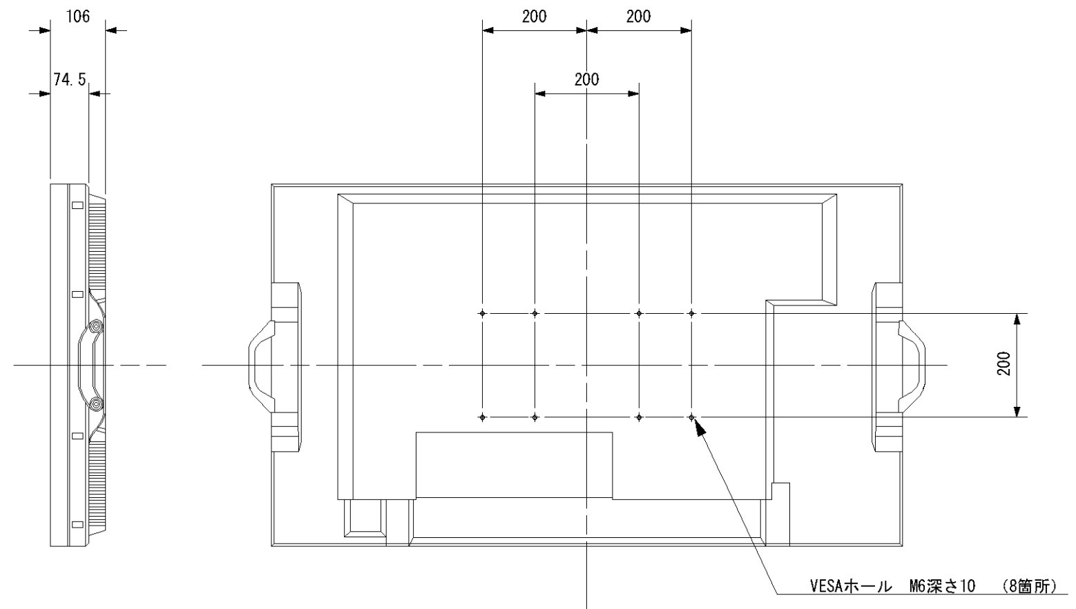
ディスプレイ 本体外観寸法図 (S=1/10)
